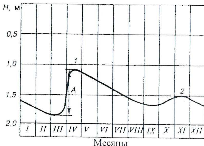
Рис.1. График колебания уровня грунтовых вод в течение года
